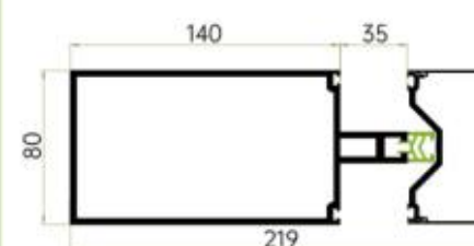
80X140断桥立柱
