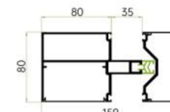
80X80断桥横梁
