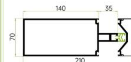
70X140断桥立柱
