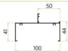
JH-PK1001 配压线JH-PK5009 100外框 | 100 Outer Frame 壁厚THK: 1.2 MM 米重W/M: 0.805 KG/M
