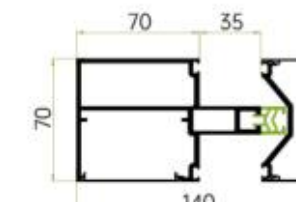
70X70断桥横梁
